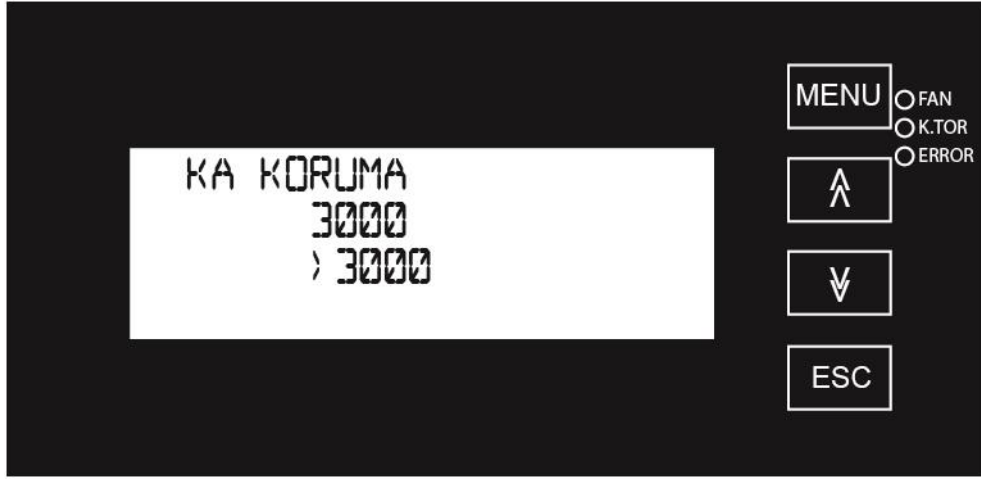
Resim21: Büyük yükte demirajı bekleme zamanı ayarı
