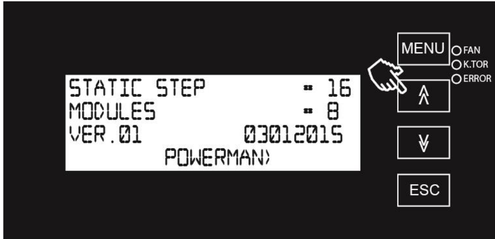
Resim7: Yukarı ok tuşuna basılınca LCD Panelde görüntülenen bilgiler
