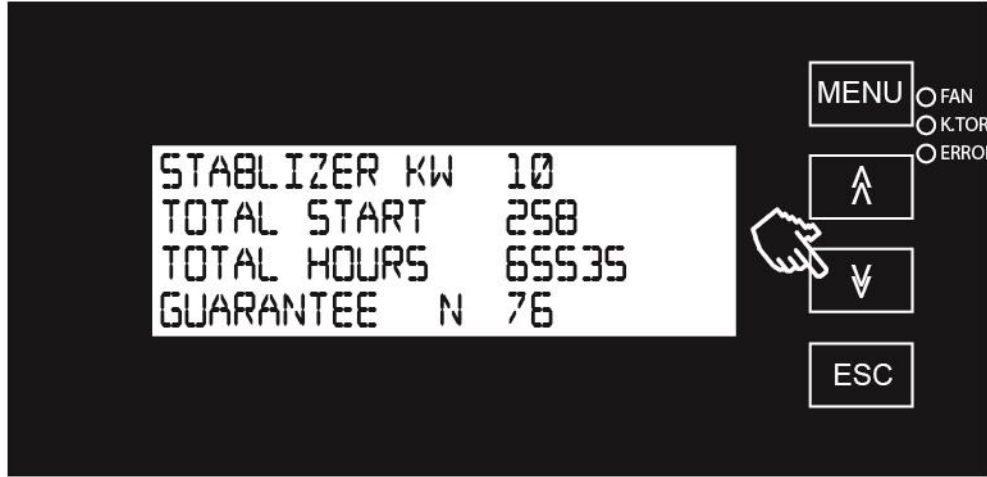
Resim8: Aşağı ok tuşuna basılınca LCD Panelde görüntülenen bilgiler
