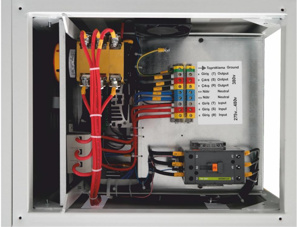
STATİK VOLTAJ REGÜLATÖRÜ 45KVA 3 FAZ ÜSTTEN GÖRÜNÜMÜ VE GİRİŞ-ÇIKIŞ KABLO BAĞLANTILARI
